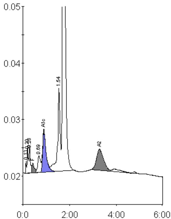
Peak table - ID: 10682546
